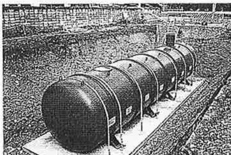
耐震性貯水槽
